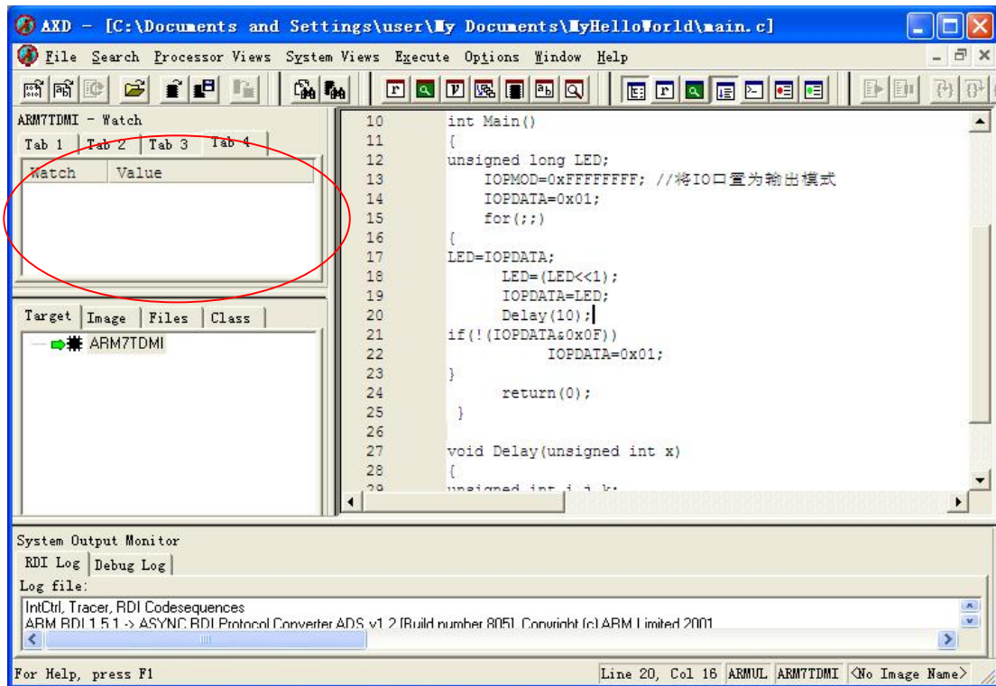
图 11.10 查看变量
