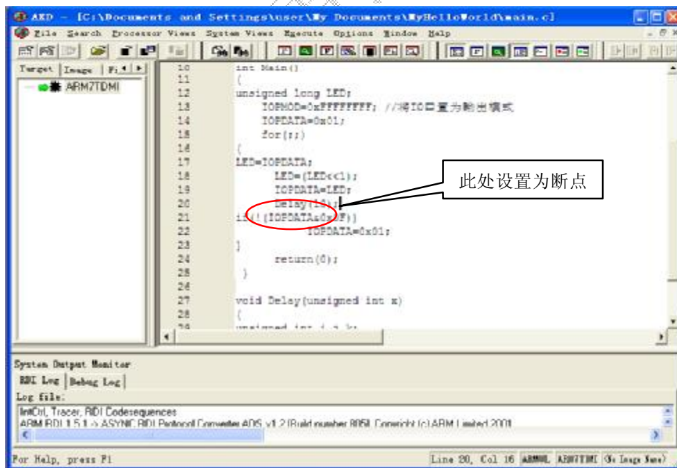
图 11.9 设置断点
